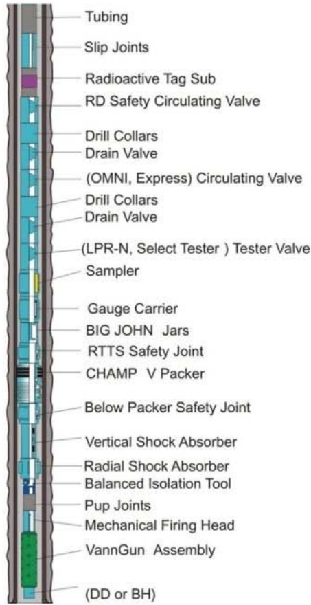
▲ DST测试工具管柱/DST Tools String
